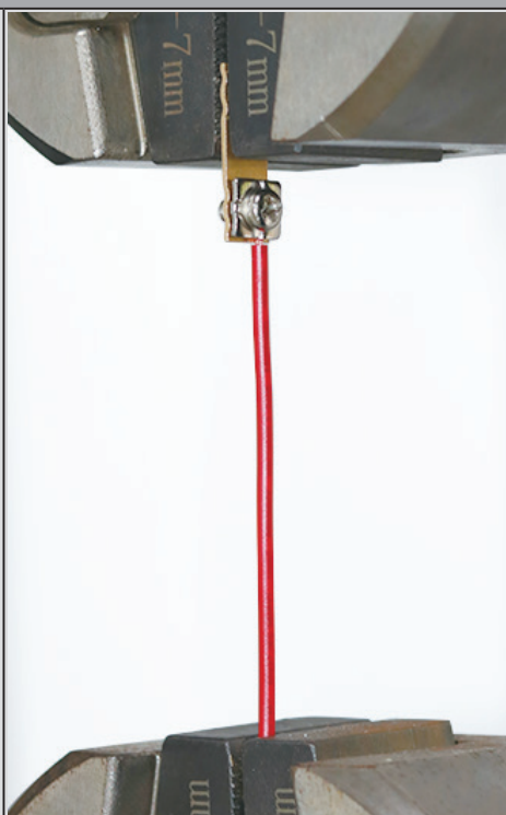
Klemmbacken-Detail
