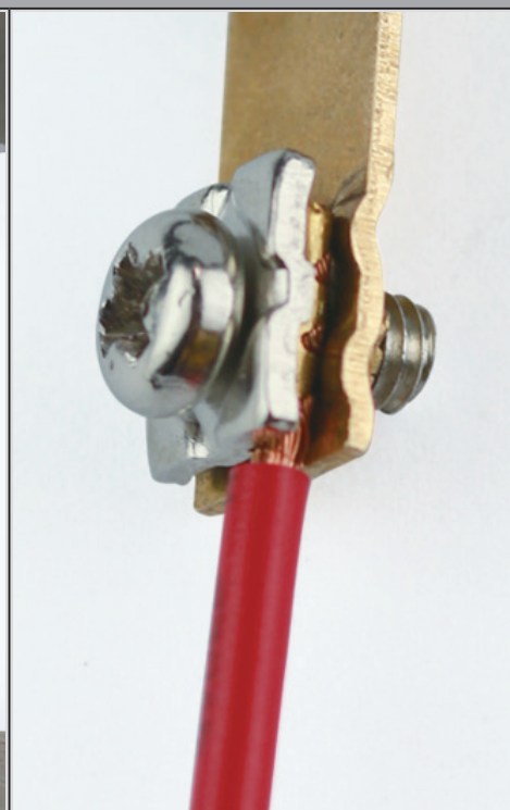
Klemmen-Detail
