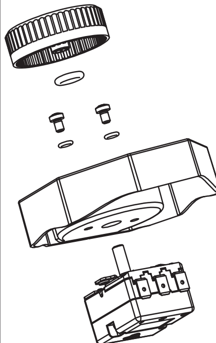
Gehäuse mit äußerem Thermostatkopf IP69K
