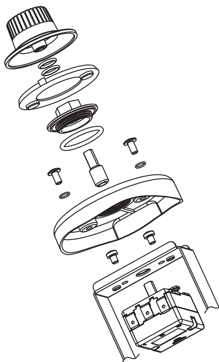
Gehäuse mit externem IP69K-Thermostatkopf
